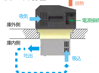
冷却ユニット模式図
