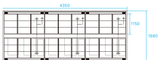
天面図
